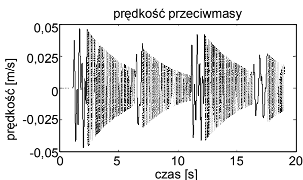
Rys. 5: Prędkość przeciwmasy
